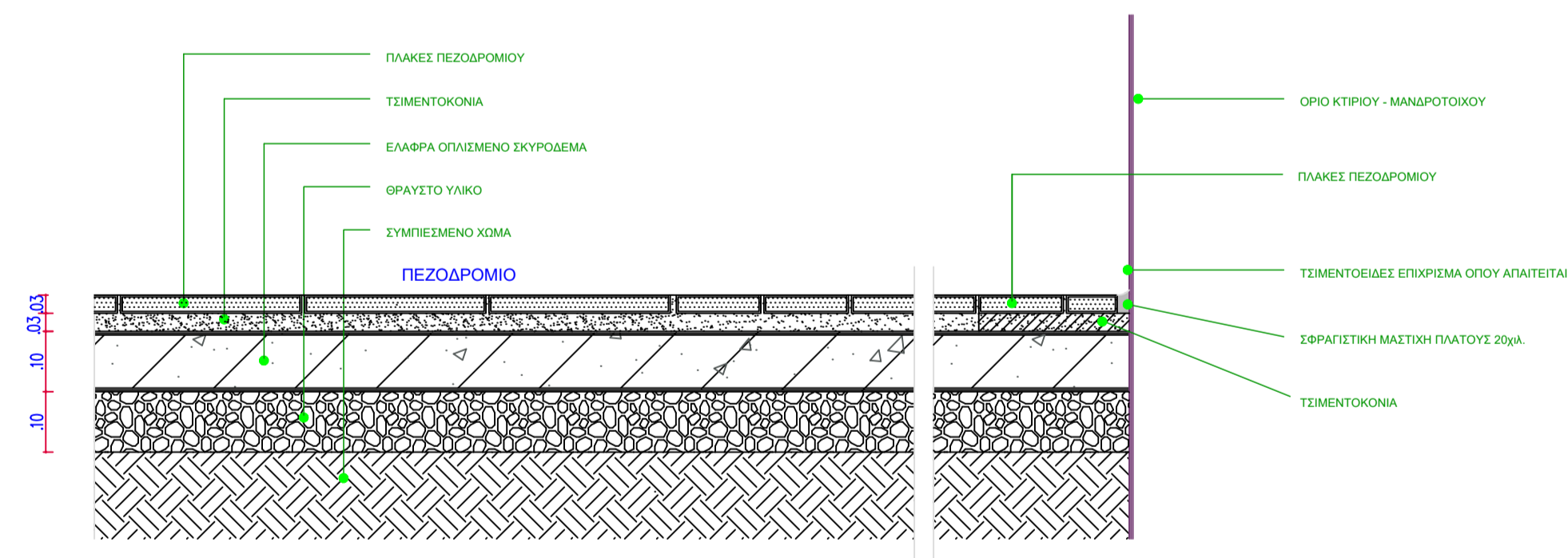
L02 - κλ. 1:10
