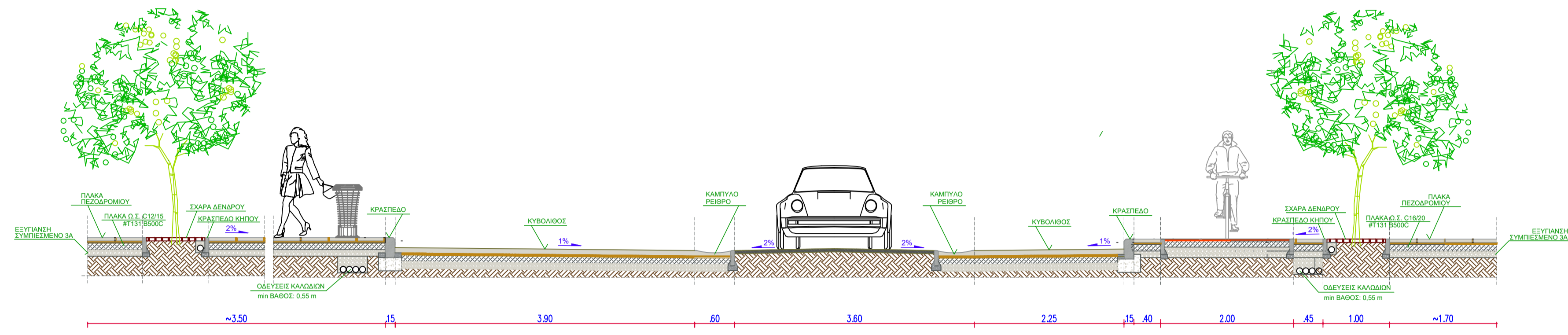
ΤΥΠΙΚΗ ΔΙΑΤΟΜΗ κλ. 1:50
