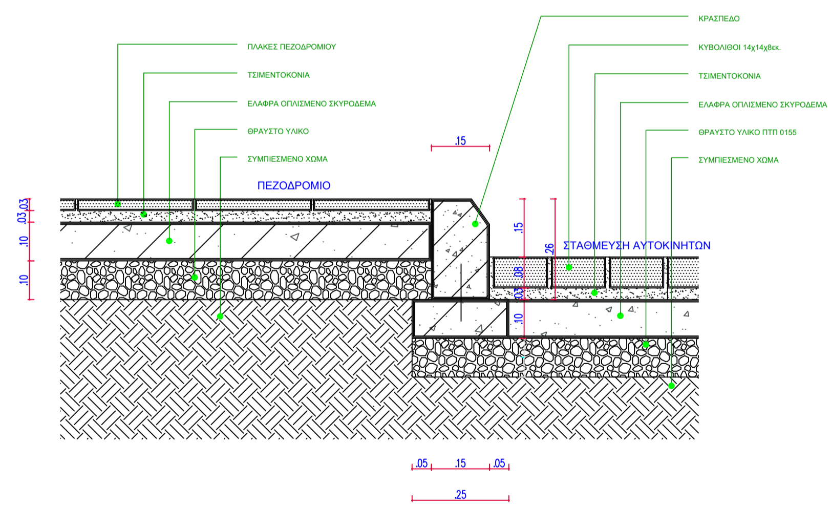
L01 - κλ. 1:10
